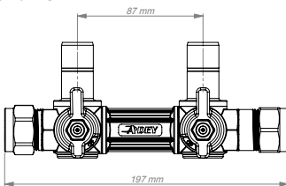
Inlet/outlet valve
